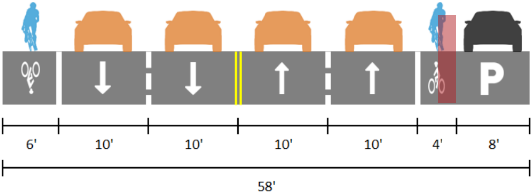
Fabian Way looking east, towards US 101 | Calle Fabian Way mirando hacia el este, hacia US 101 Door Zone | Zona de las puertas
