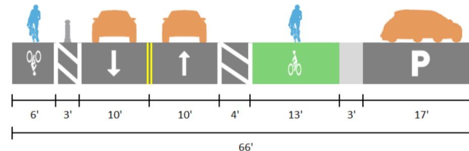
Option 2 Protected Bike Lanes | Opción 2 Ciclovías
