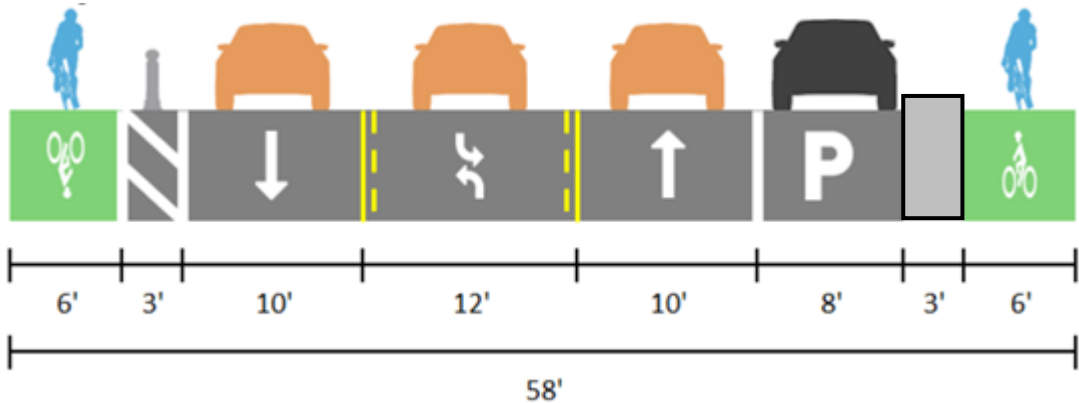
Option 2 Protected Bike Lanes | Opción 2 Ciclovías
