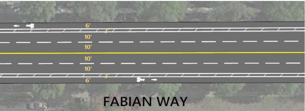
Potential Layouts | Posibles Diseños
